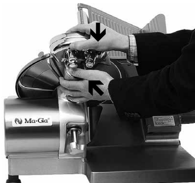
Rys. 8. Przesuwanie do ostrzenia
