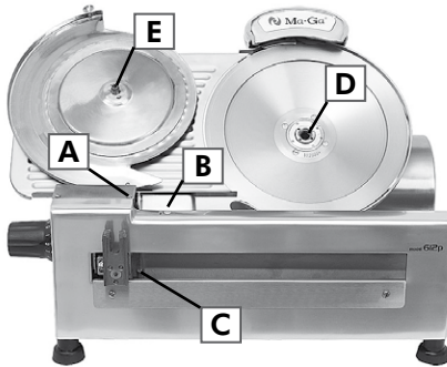
Rys. 14. Punkty smarne
